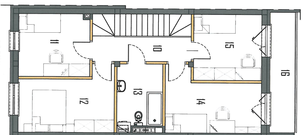
RZUT PIĘTRA
