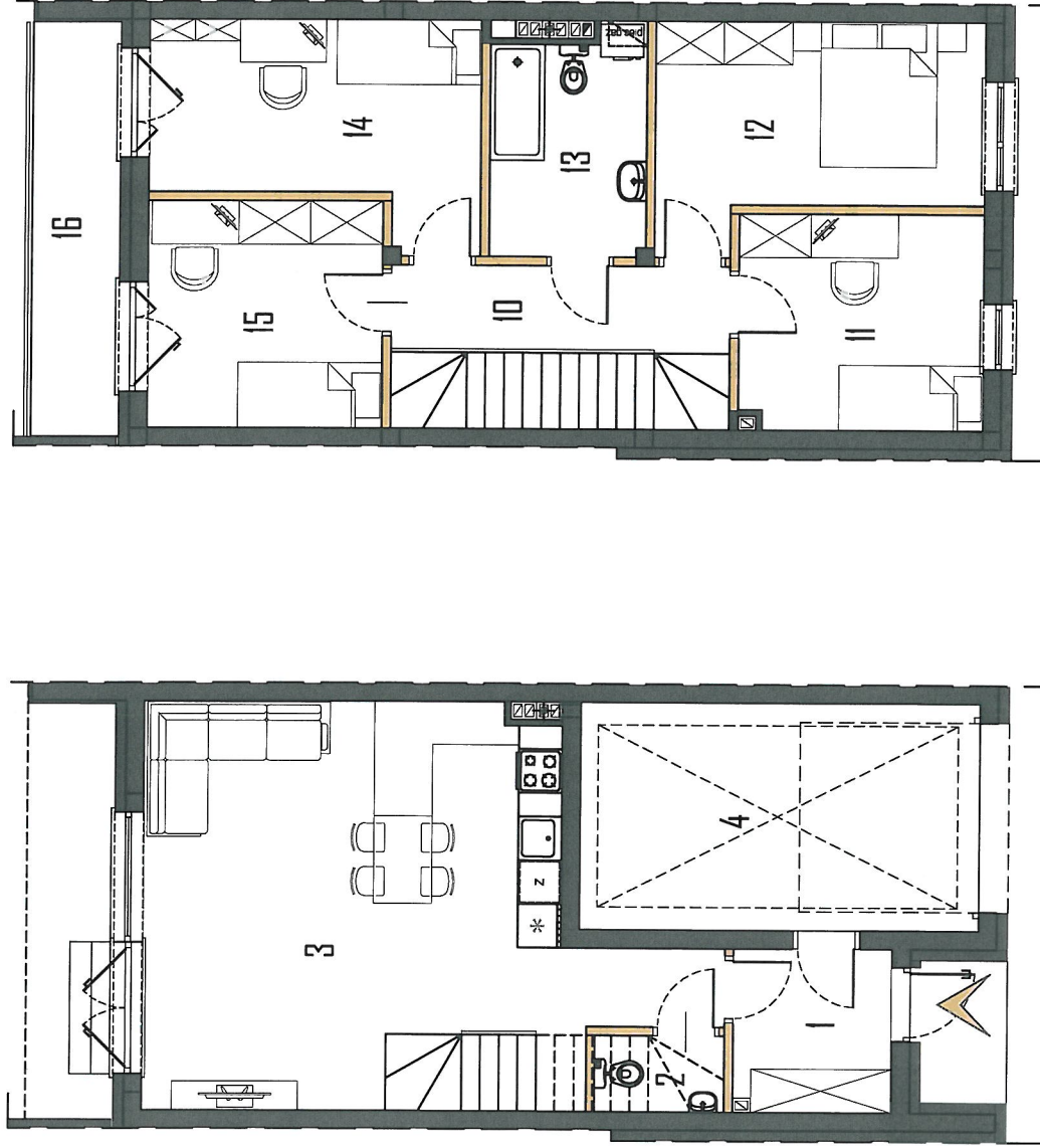
RZUT PARTERU
