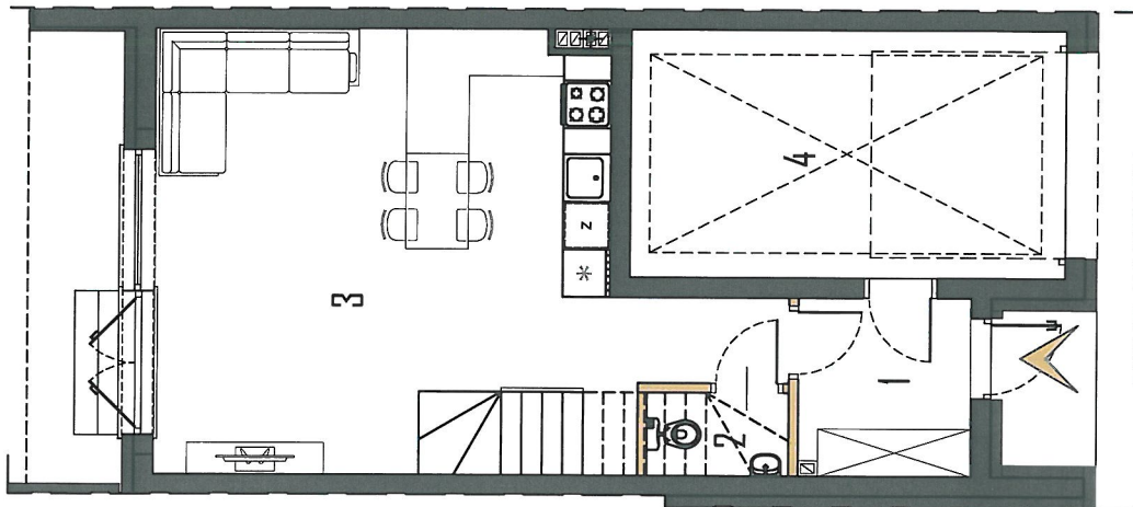
RZUT PARTERU
