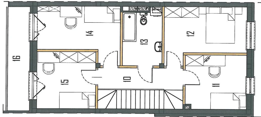
RZUT PIĘTRA
